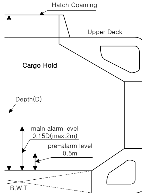
그림 1 선박깊이(D)
